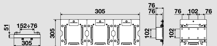
Art. 843013 Staffa per il montaggio di 3 avvolgitubo s. 390 o 430 su trave HEA.
